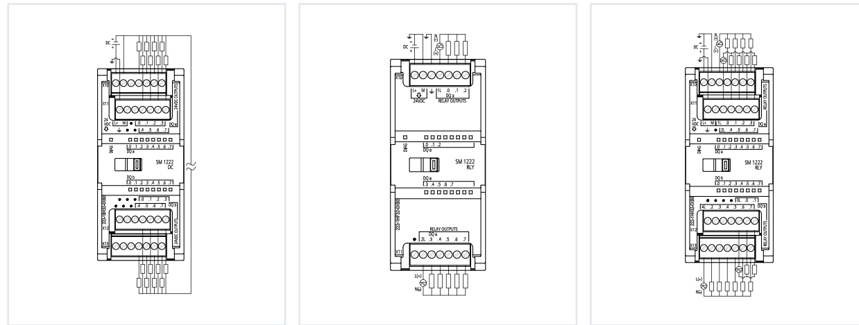
Article No.: H7-222-1BH32-0XB0 Model numbe: SM 1222 DQ 16x24 V DC
